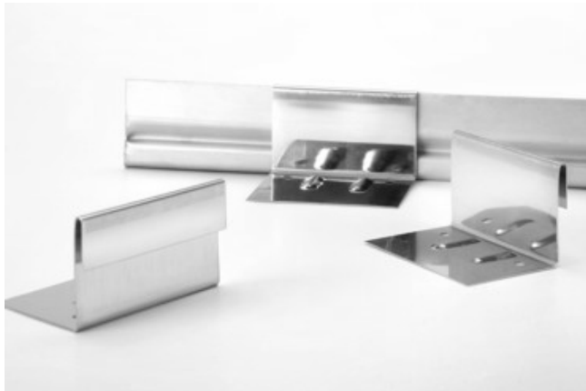
Ausführung für Falzhöhe 38 mm
